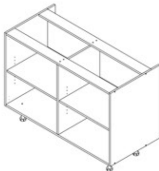
ELEMENT BAS POUR 2 PORTES
